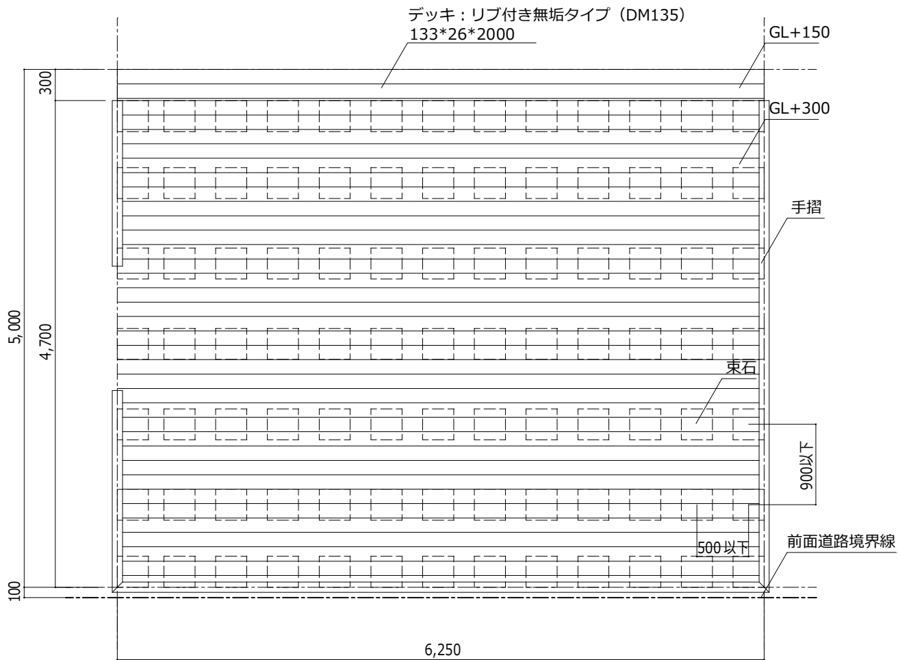
平面図
